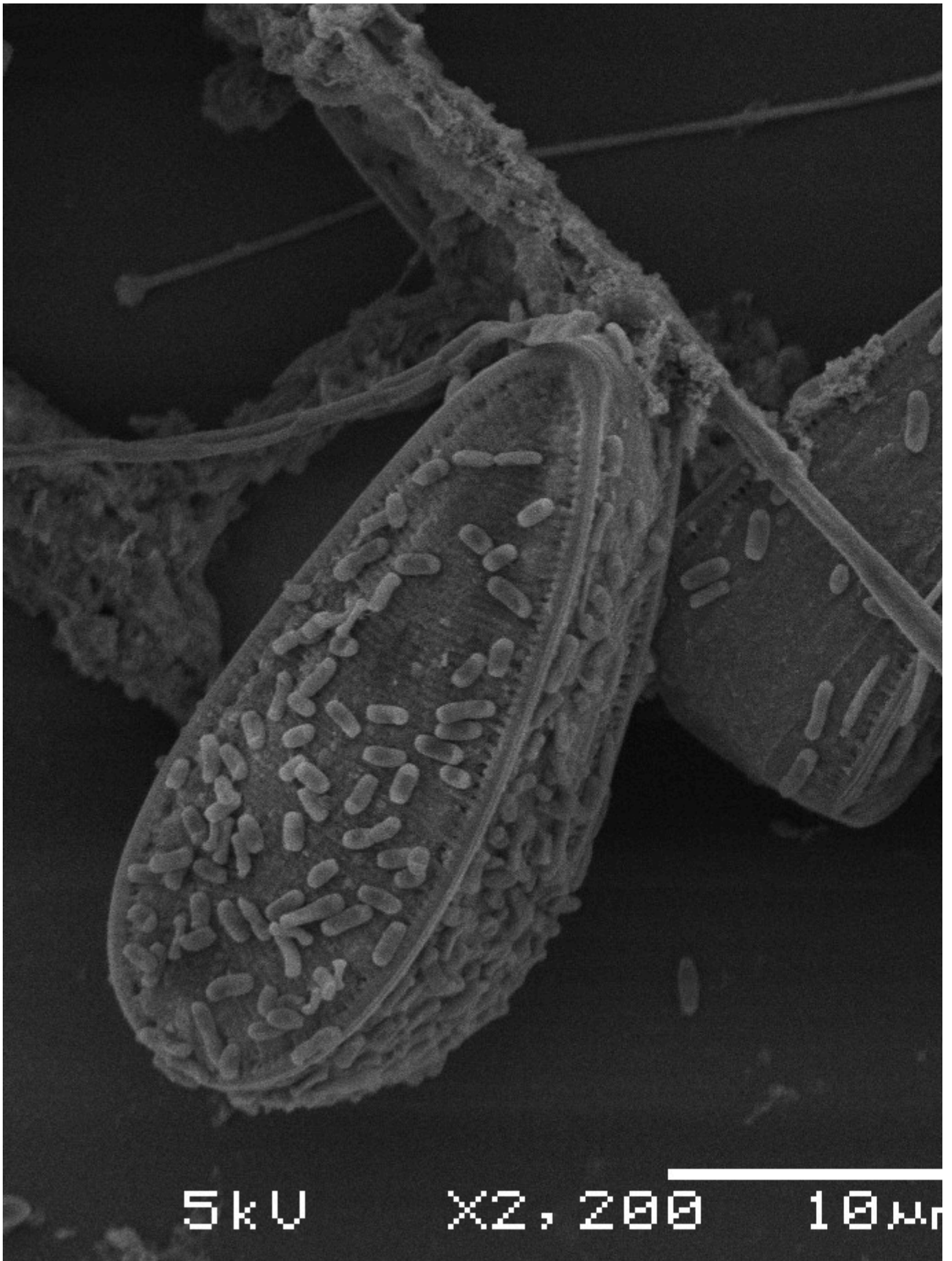
Diatomées
